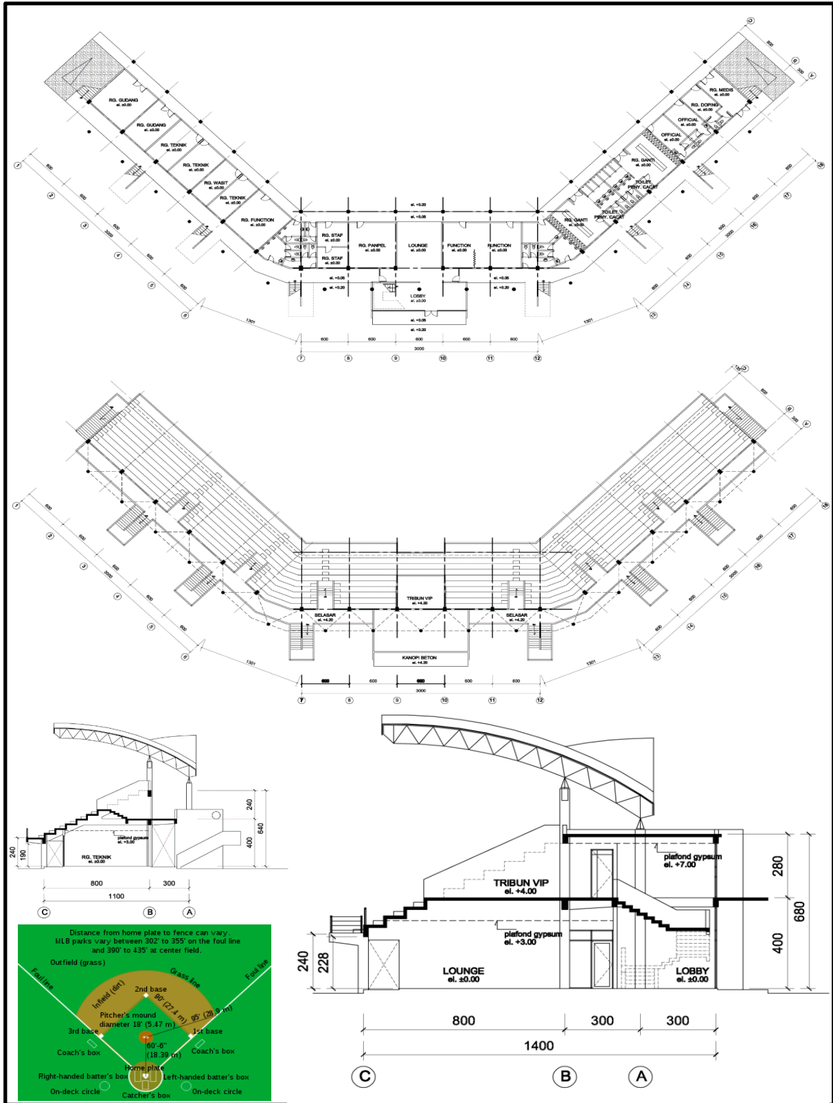
GAMBAR TEKNIS DALAM - LUAR DAN HALAMAN GEDUNG
