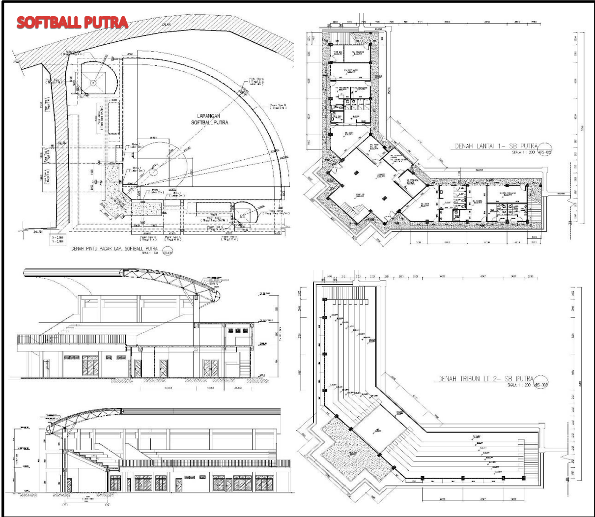
GAMBAR TEKNIS DALAM - LUAR DAN HALAMAN GEDUNG
